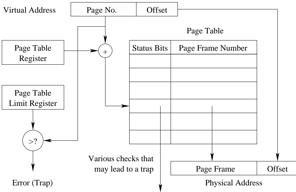
Figure 3. Pure Paging
